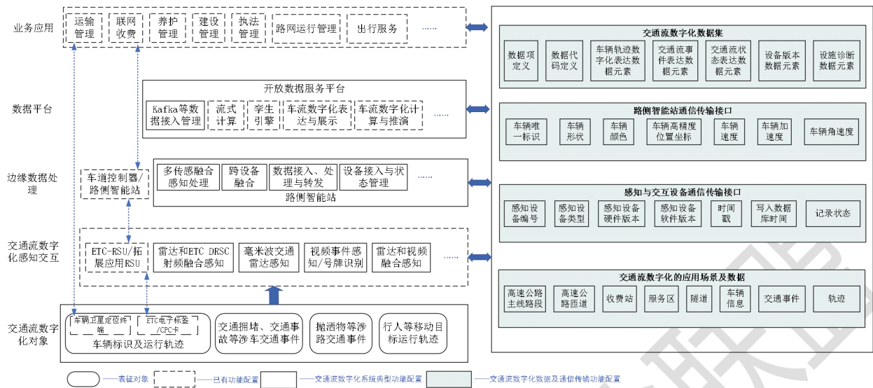
图1 交通流数字化相关智慧公路系统功能框架图
