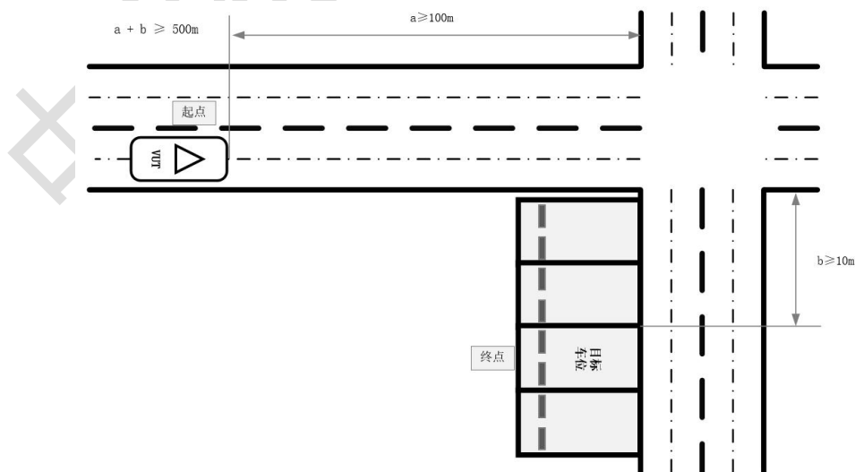
图 2 学习建图试验场景示意图
