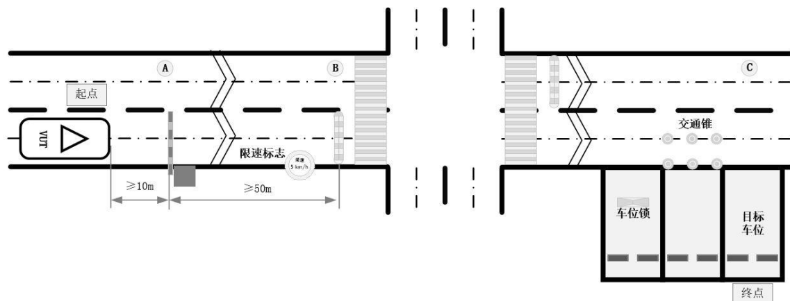
图 6 道路设施的探测与响应试验示意图
