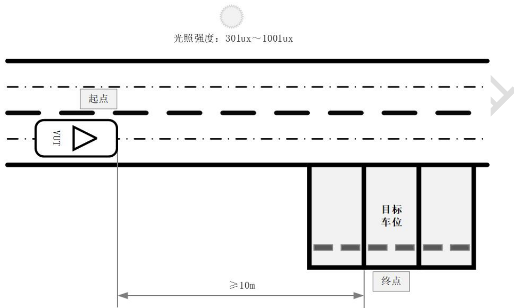
图4 泊车环境（光照强度）适应性试验示意图
