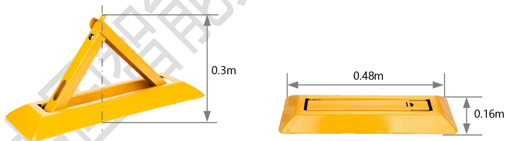
图 A.2 车位锁示意图
