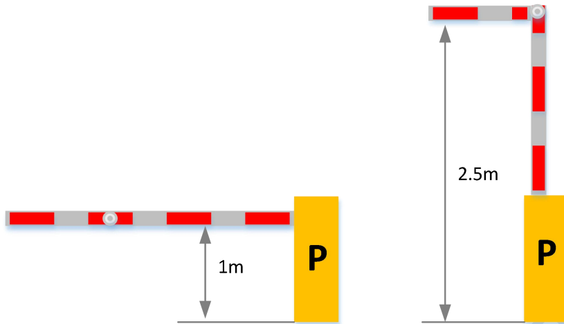
图 A.3 收费杆示意图
