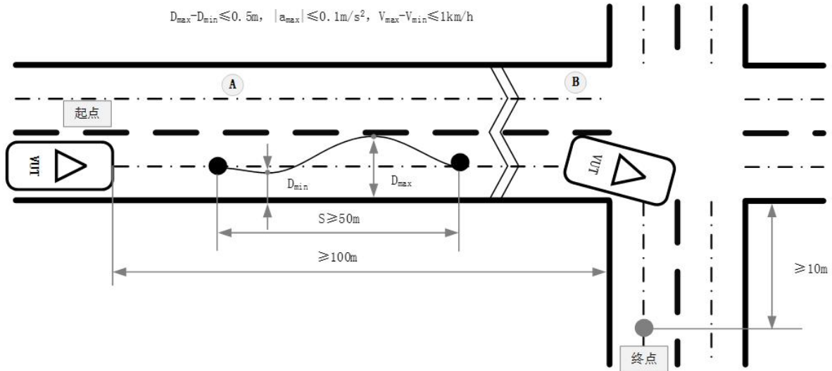
图 3 道路结构适应性试验示意图
