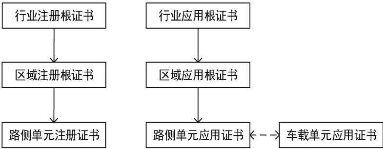
图2 路侧单元与车载单元间证书体系
