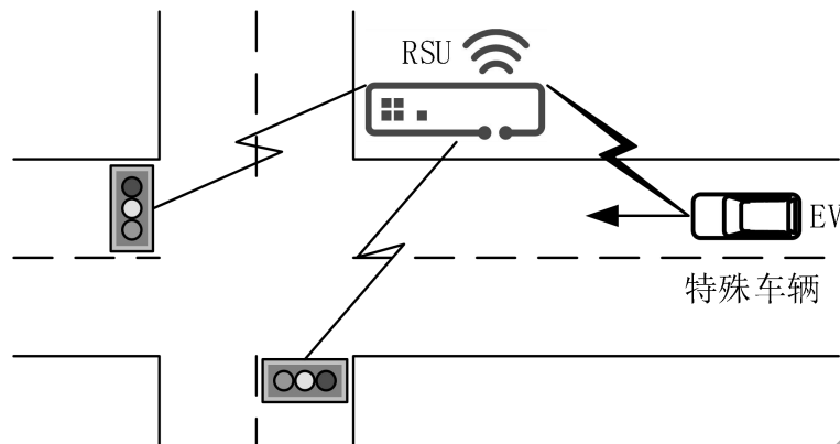
图 20 RSU 协调信号灯优先通行
