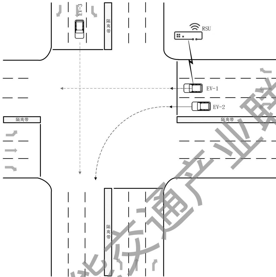
图 14 RSU 辅助车辆通过无信号灯路口
