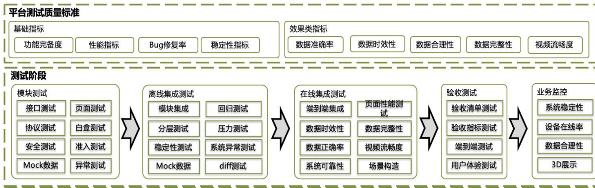
图1 云控平台测试体系架构
