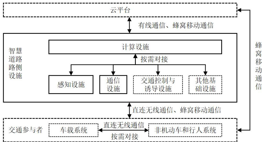
图 1 车路云一体化路侧基础设施架构
